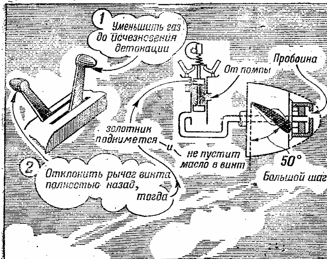
Рис. 23 Полет с поврежденной маслосистемой ВИШ прямой схемы (ВИШ-21, ВИШ-22, ВИШ-23, ВИШ-105)
