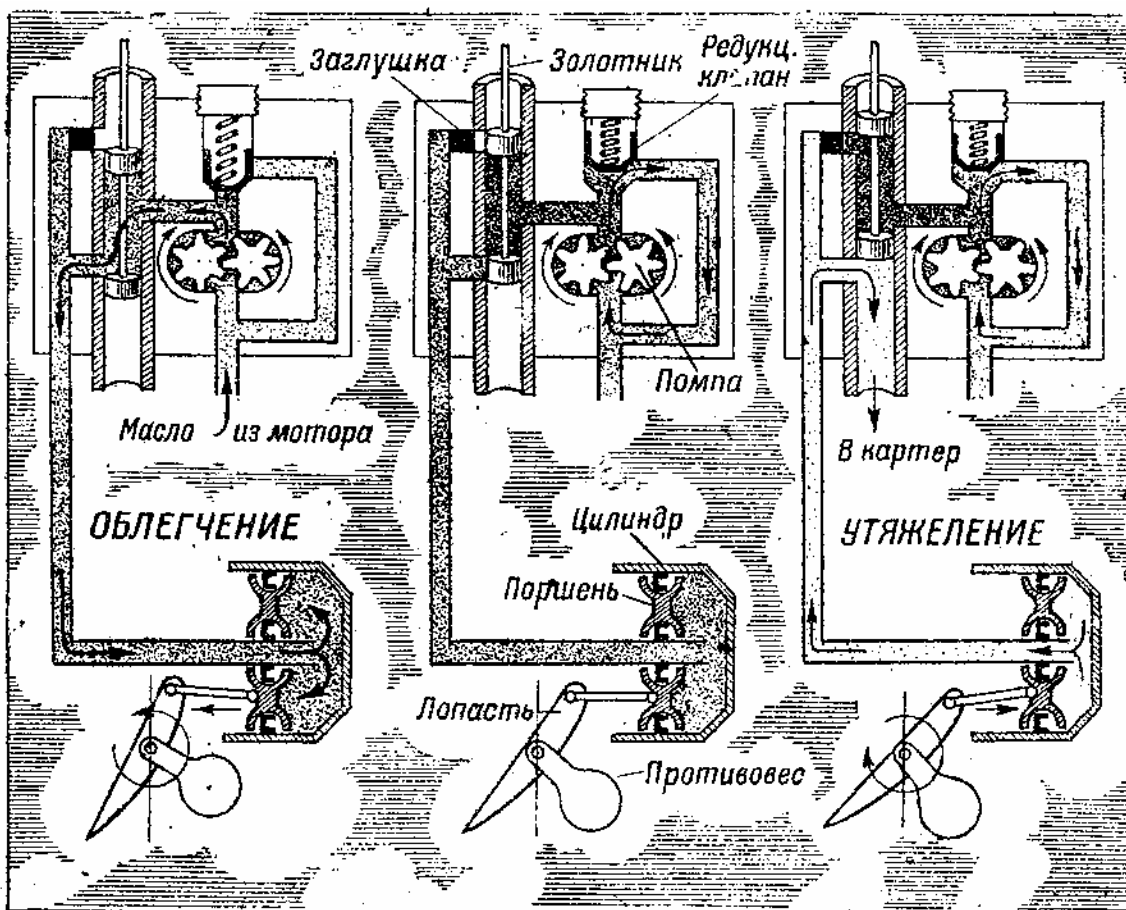
Рис. 12 Работа гидросистемы винта прямой схемы
