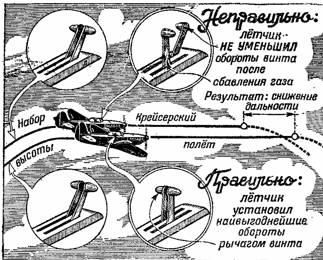
Рис. 21 Увеличение дальности полета применением наиболее выгодных оборотов
