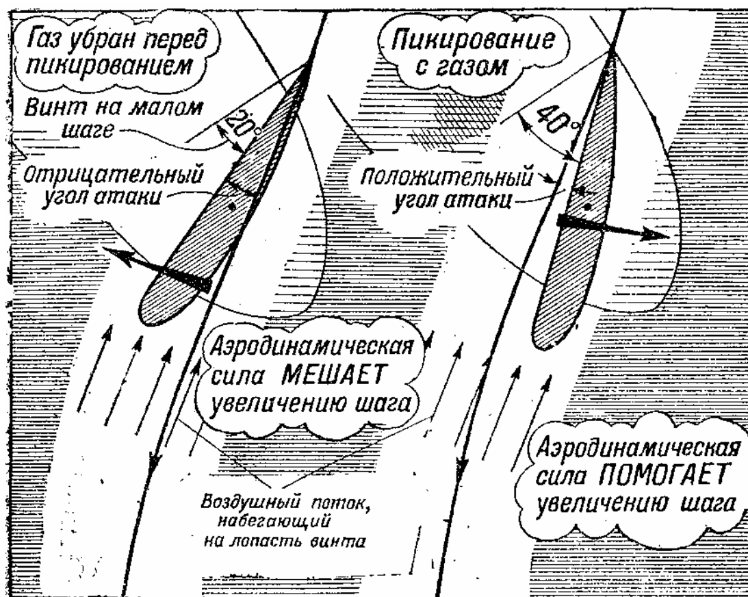
Рис. 26 Раскрутка атоматического ВИШ вследствие полной уборки газа перед вводом в пикирование
