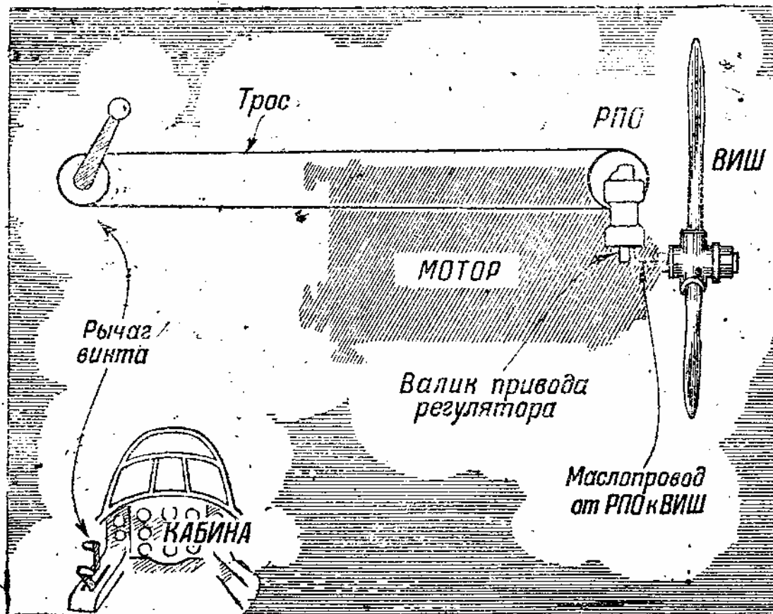
Рис. 11 Принципиальная схема установки автоматического винта на самолете
