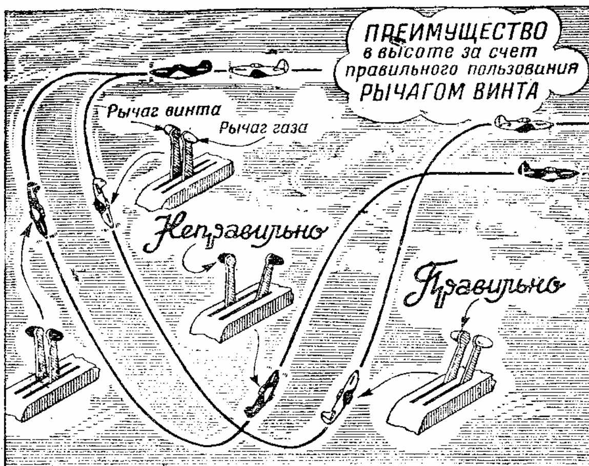
Рис. 27 Пользование рычагом винта при вертикальном маневре
