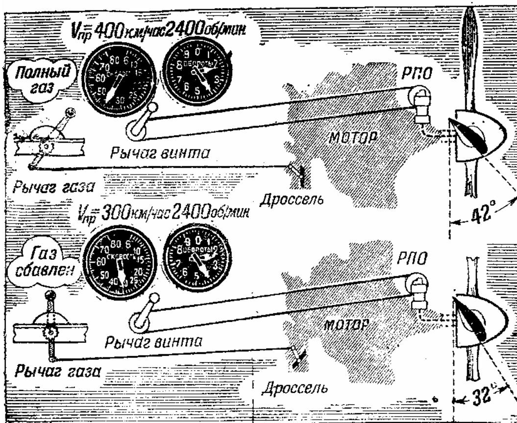
Рис. 16 Изменение шага автоматического винта, вызванное дросселированием мотора
