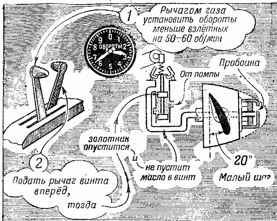
Рис. 22 Полет с поврежденной маслосистемой ВИШ обратной схемы (АВ-5, ВИШ-61)
