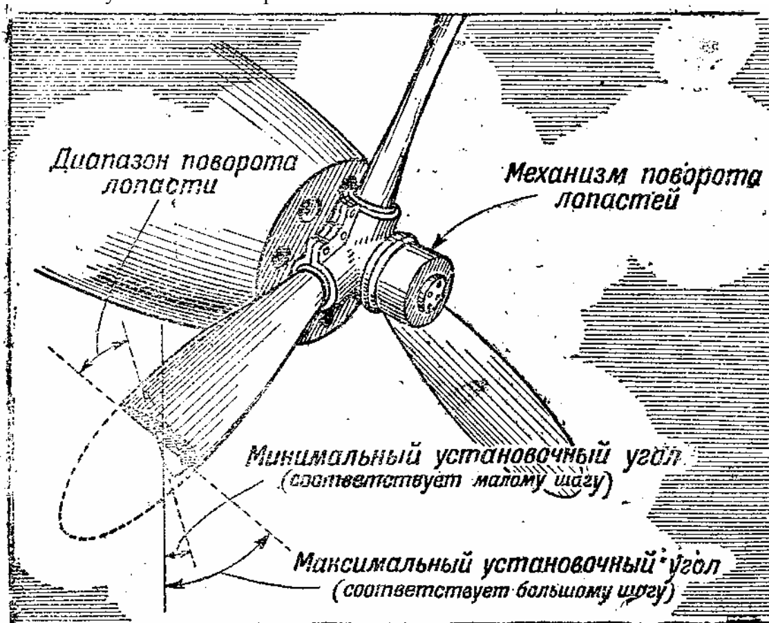
Рис. 8 Винт изменяемого в полете шага
