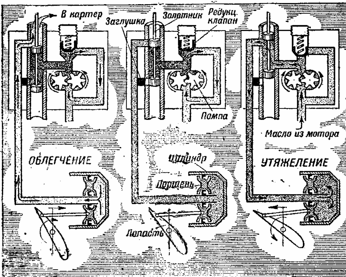
Рис. 13 Работа гидросистемы винта обратной схемы
