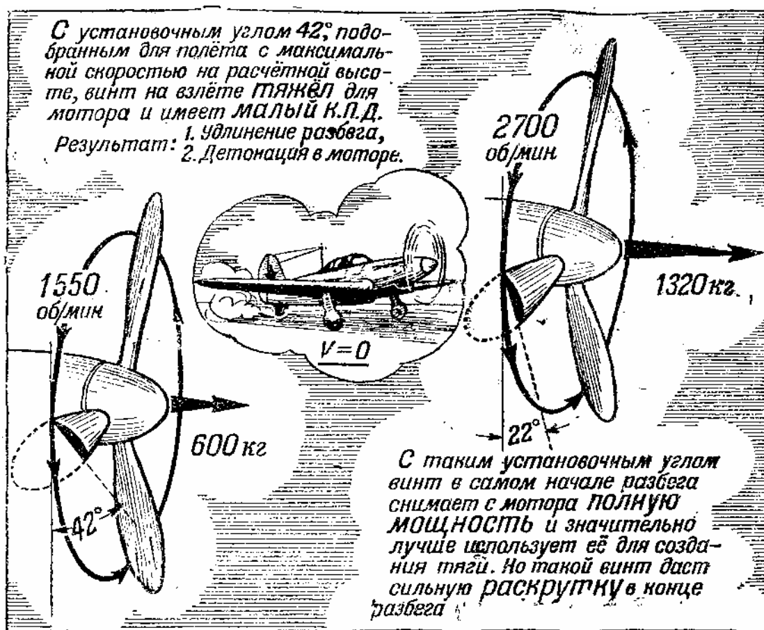
Рис. 6 Работа винта в начале разбега (полный газ)
