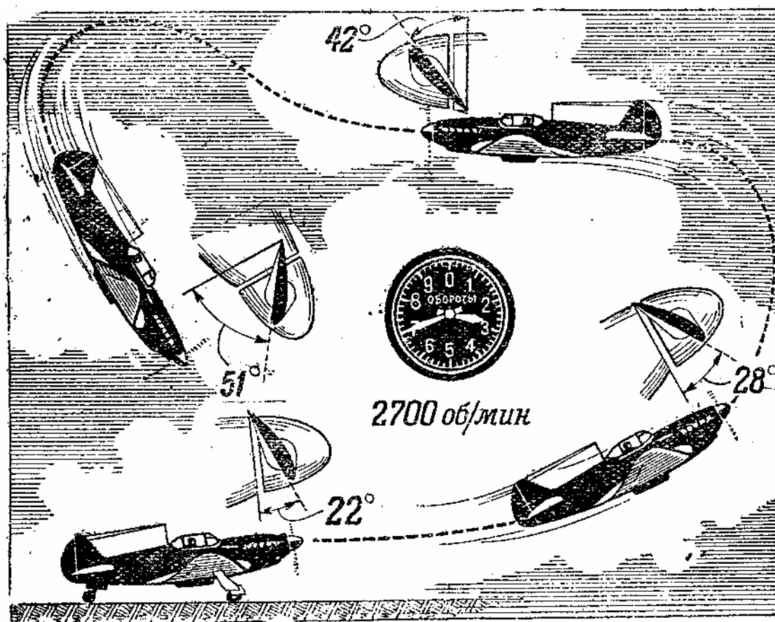
Рис. 9 Сохранение постоянных оборотов автоматическим винтом на различных режимах полета с полным газом
