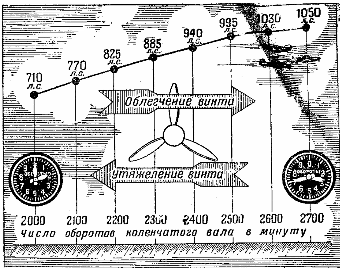
Рис. 2 Изменение мощности мотора ВК-105 на высоте 4000м (полный газ) при изменении оборотов облегчением и утяжелением винта
