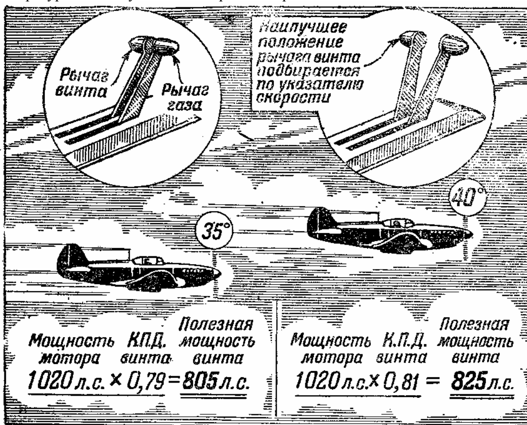
Рис. 20 Повышение максимальной скорости на высотах, меньших расчетной, за счет снижения числа оборотов рычагом винта
