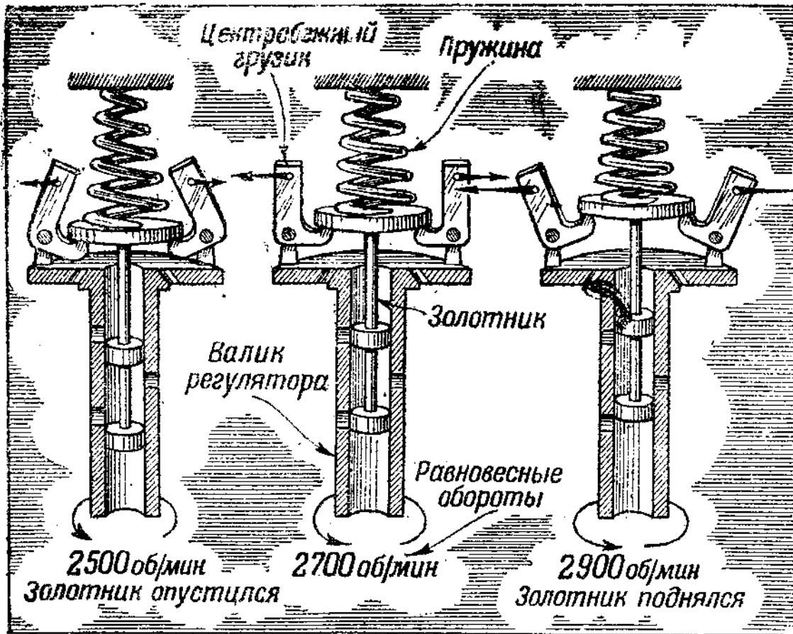
Рис. 14 Схема действия центробежного РПО
