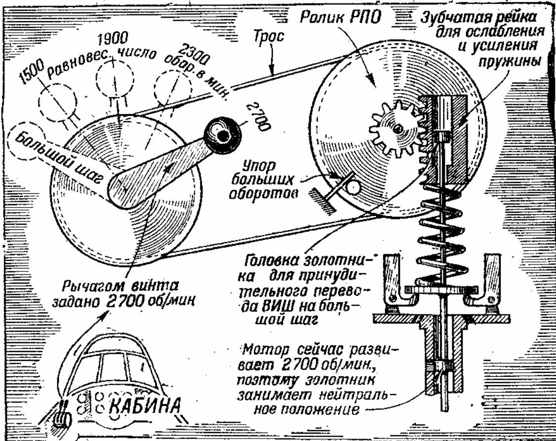
Рис. 15 Схема управления винтом из кабины летчика
