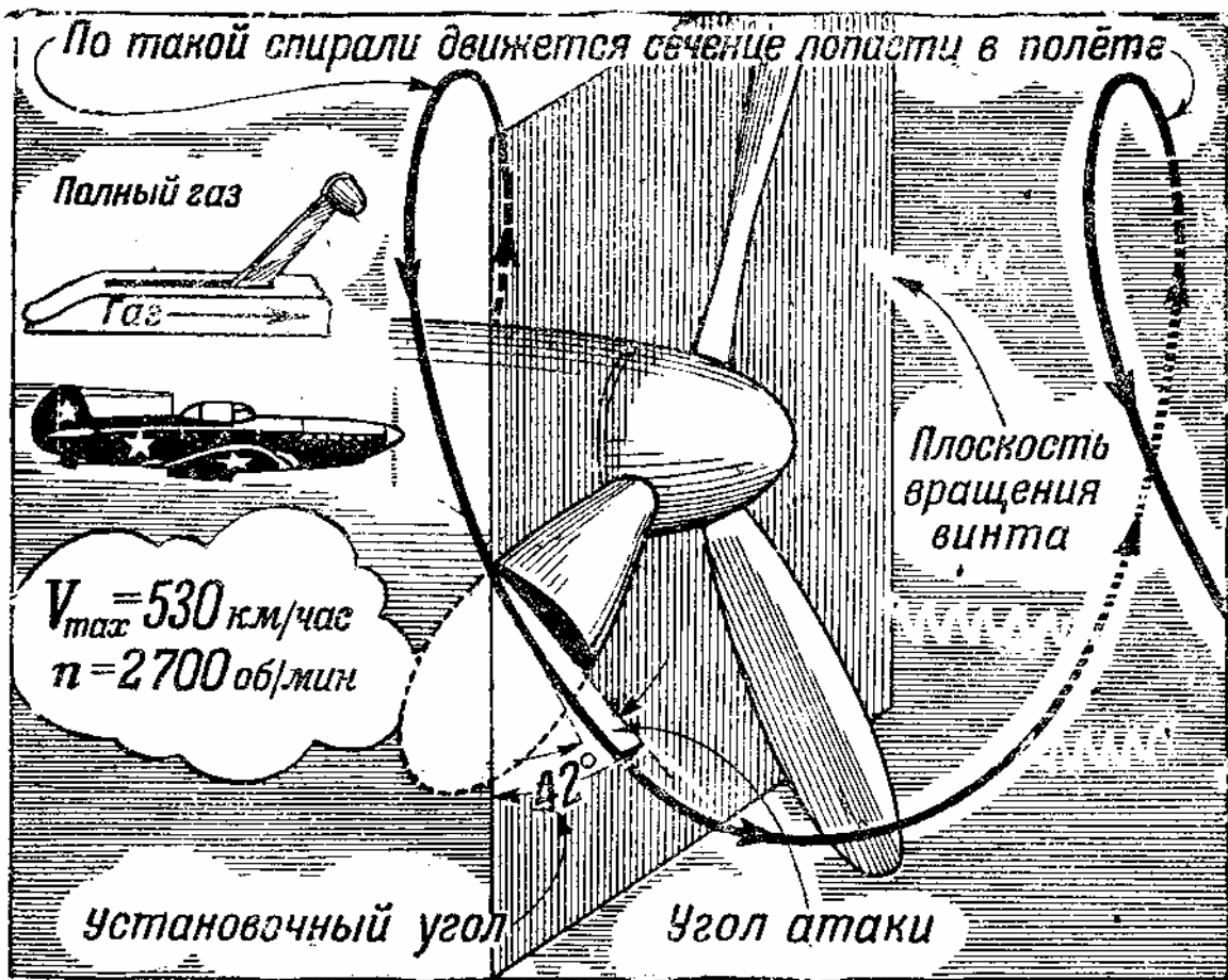
Рис. 3 Работа винта в горизонтальном полете
