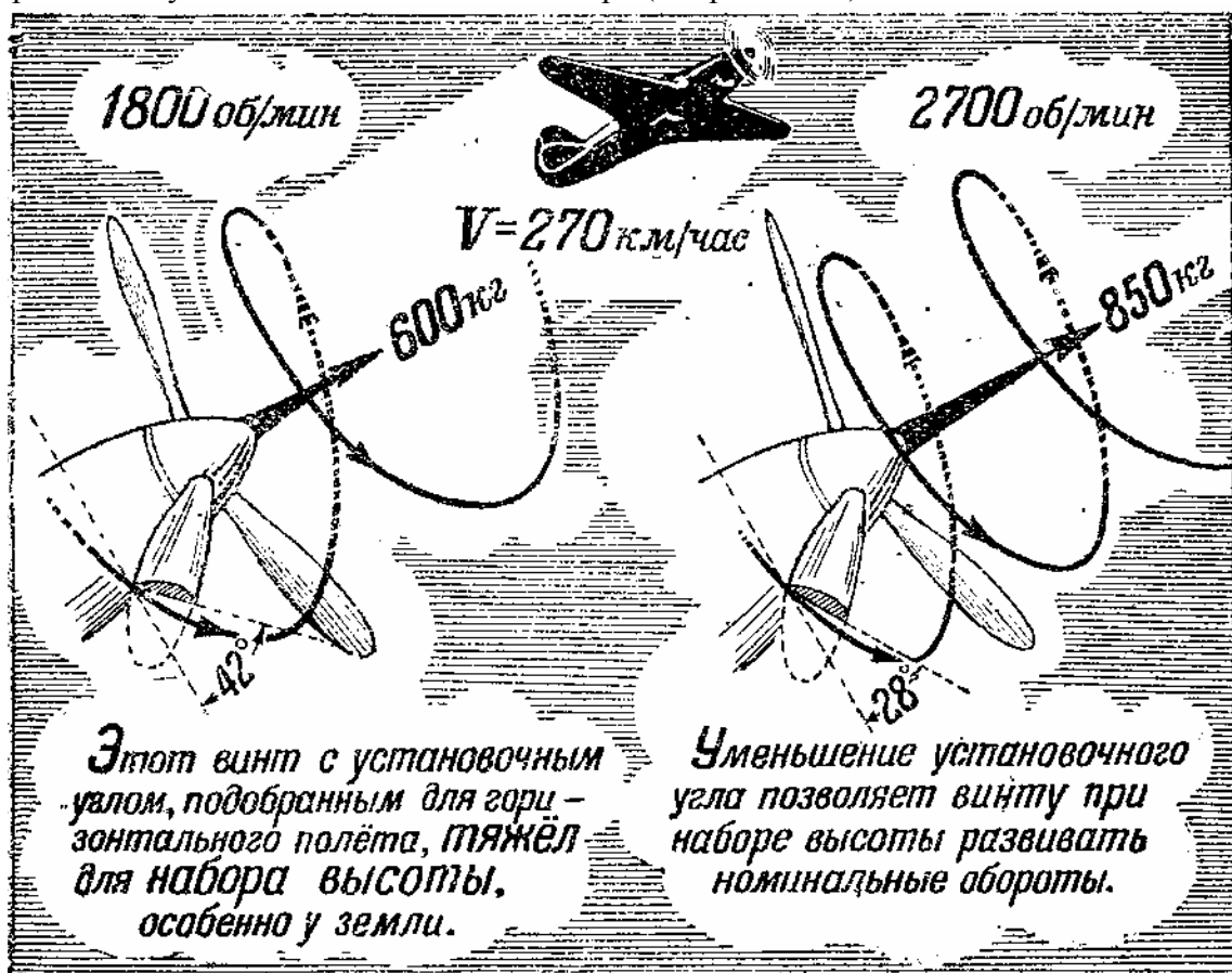
Рис. 5 Работа винта при наборе высоты (полный газ)
