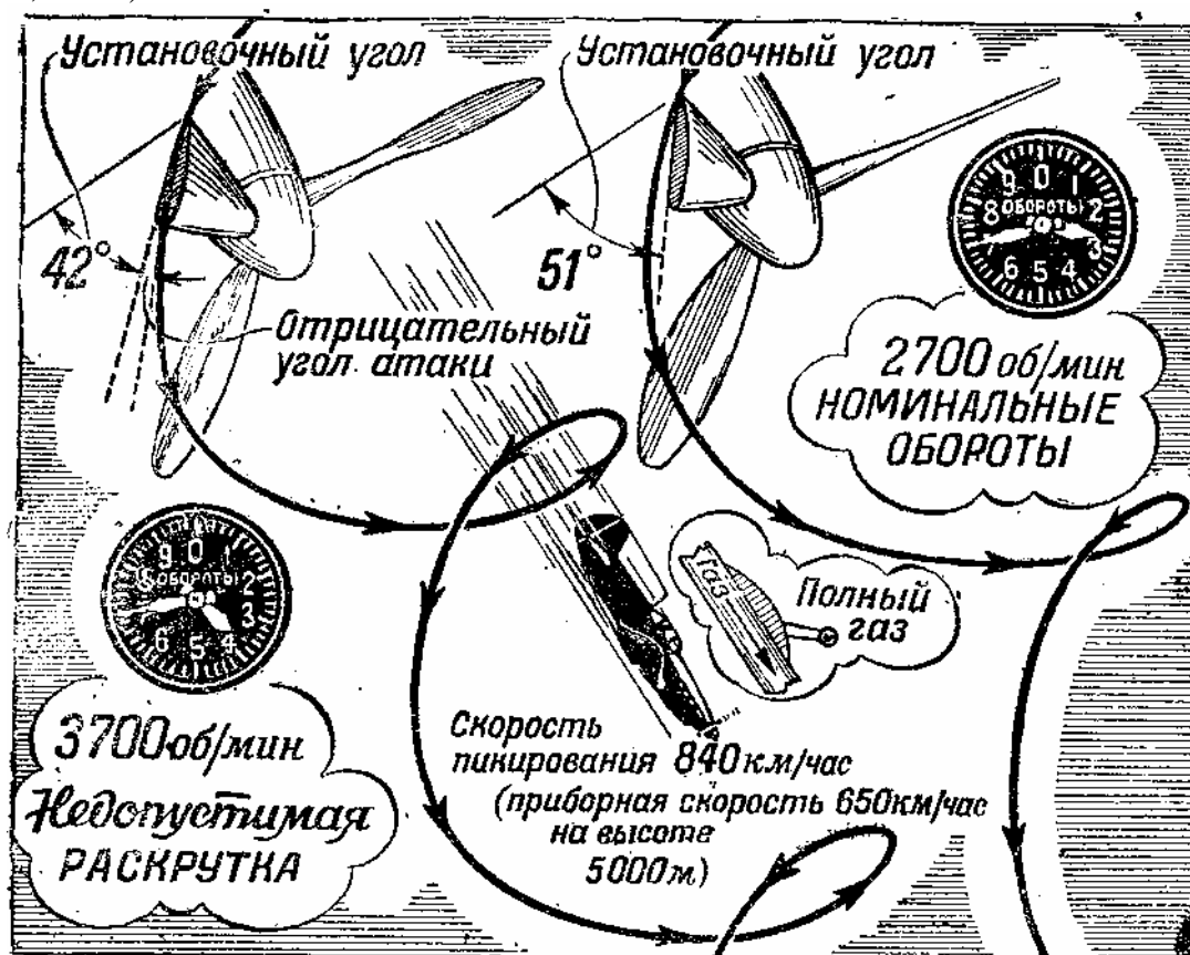
Рис. 7 Работа винта с различными установочными углами при пикировании
