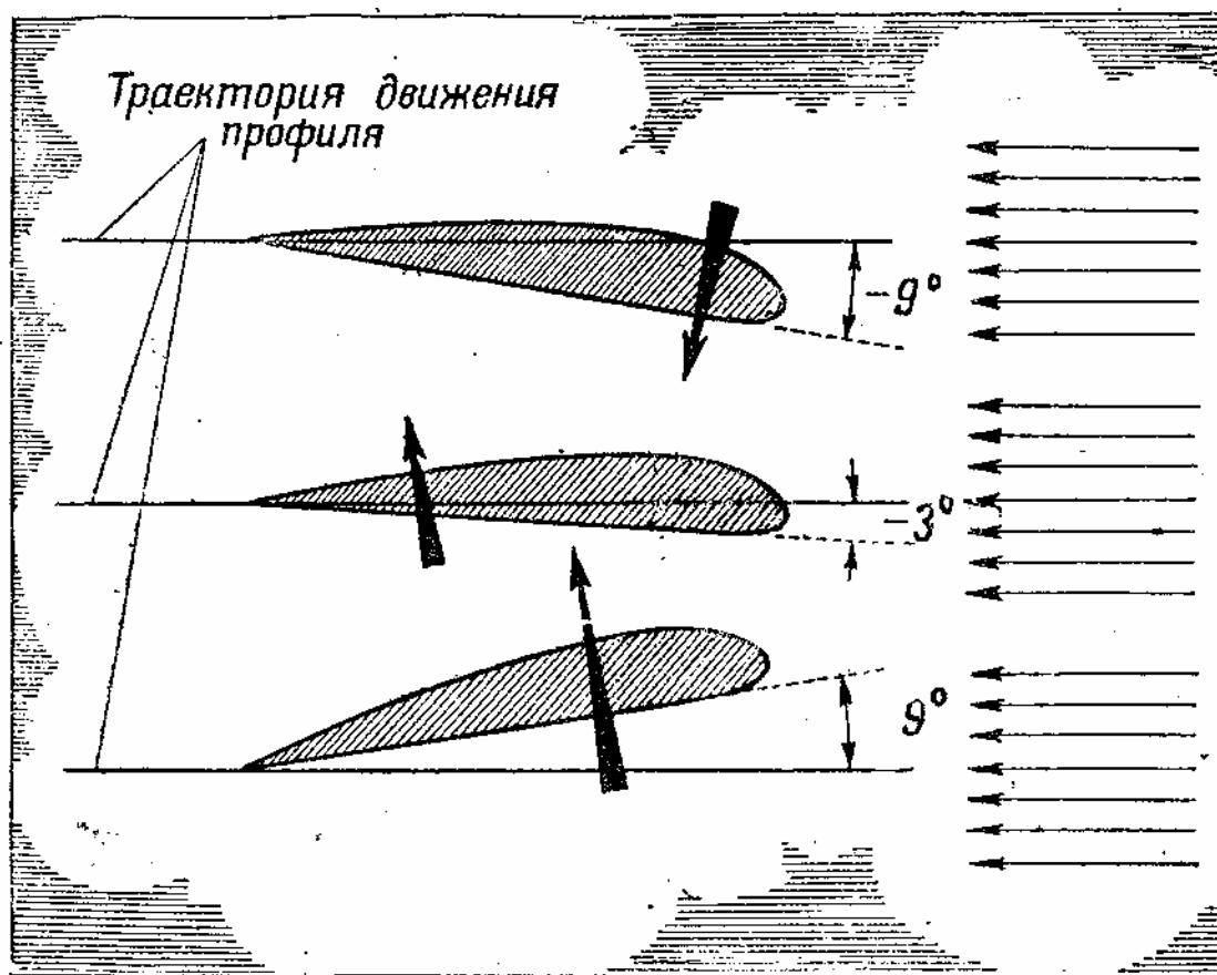
Рис. 25 Положение аэродинамической силы профиля при различных углах атаки
